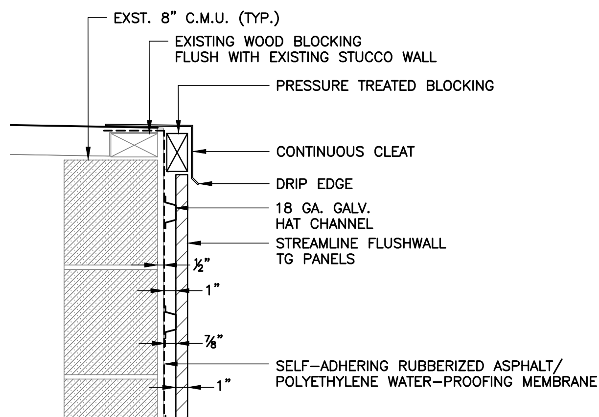
3 SECTION SCALE: 1-1/2" = 1'-0"
