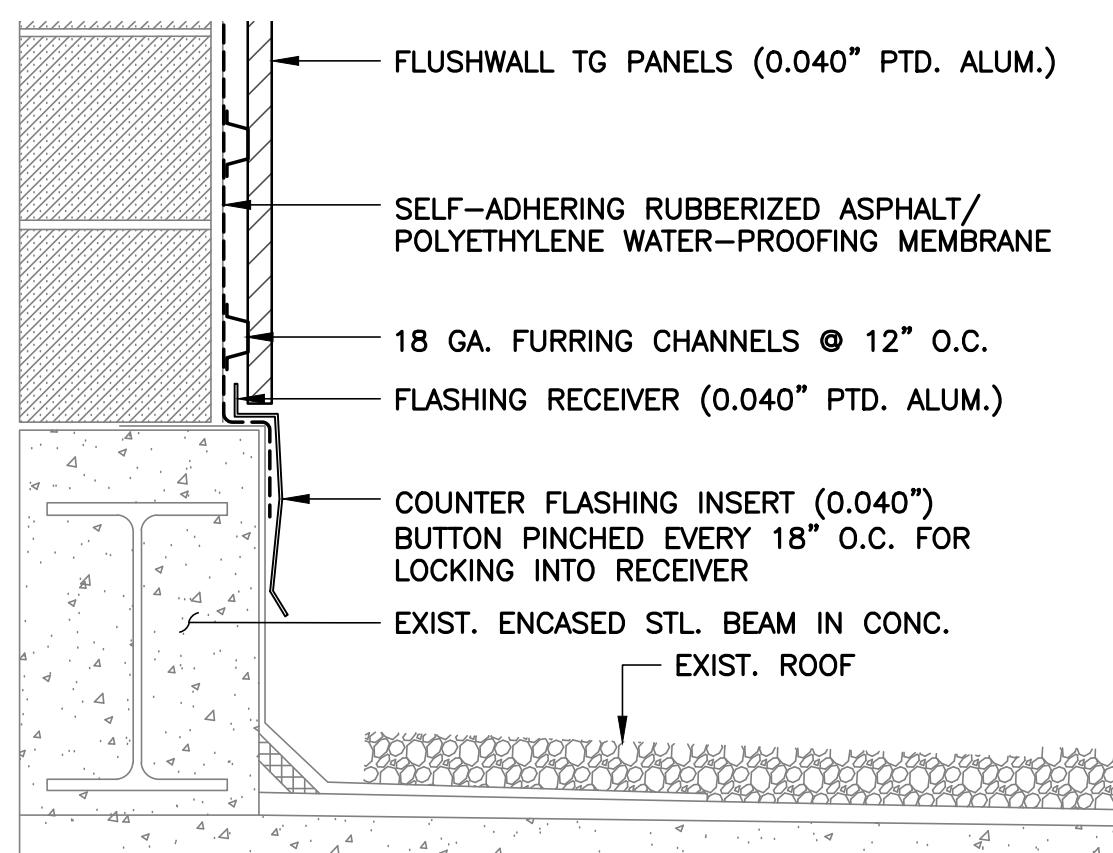
4 SECTION THRU EXISTING PARAPET SCALE: 1-1/2" = 1'-0"
