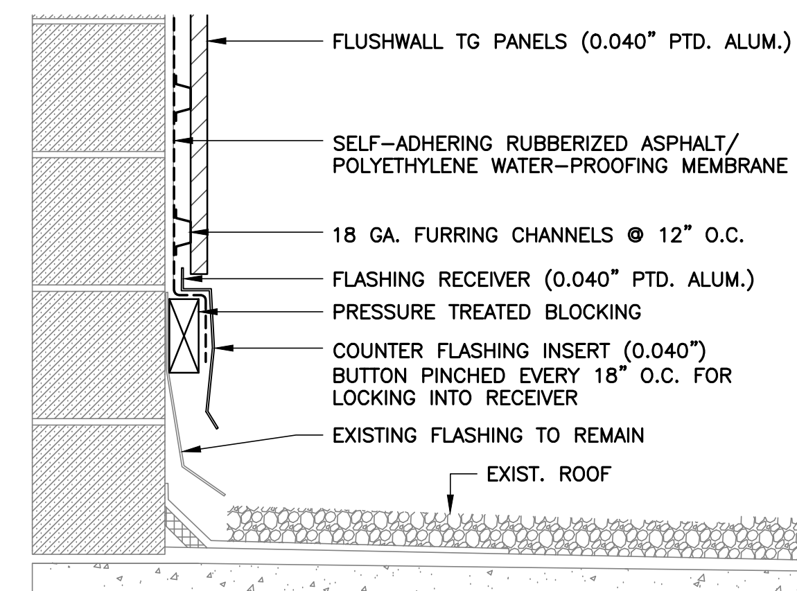
4a SECTION THRU EXISTING PARAPET SCALE: 1-1/2" = 1'-0"
